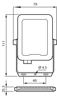
BVP164 LED12/840 PSU 10W SWB CE
